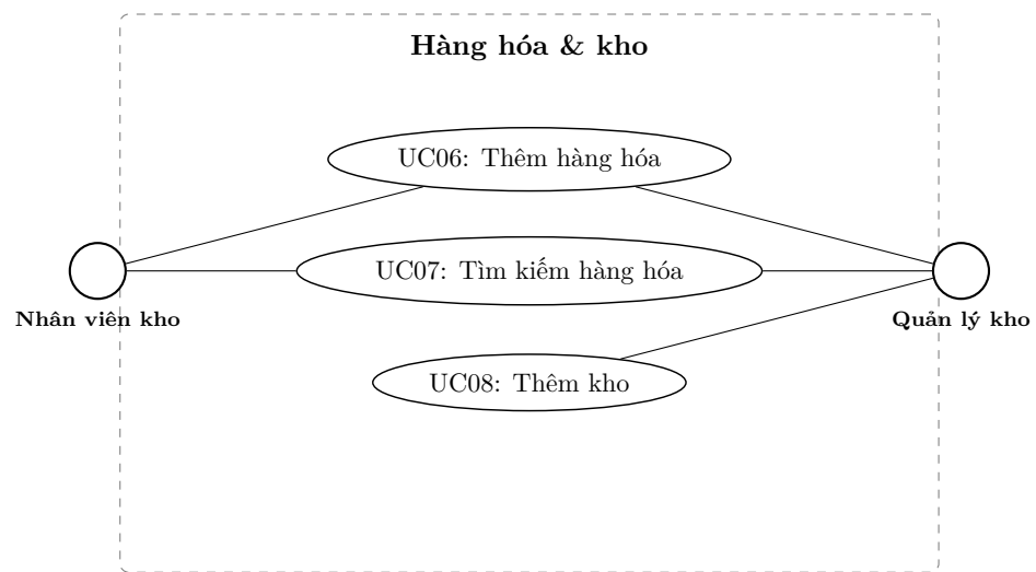
Figure 1: Sơ đồ use case phân rã – Hàng hóa và kho
